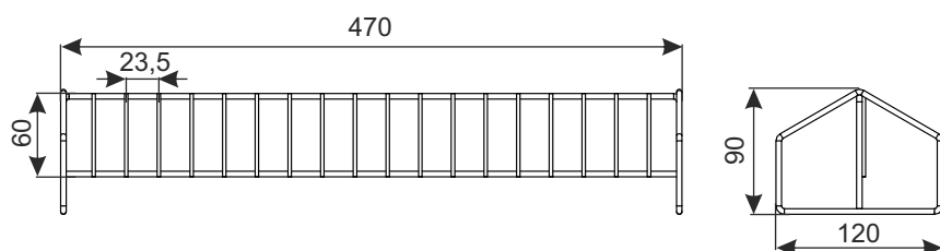
Drahtquertrennwand L-470
